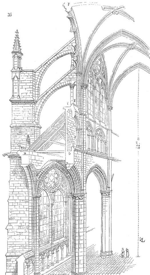
Coupe de la nef de la cathédrale d'Amiens (d'après E. Viollet Le Duc, Dictionnaire raisonné de l'architecture française du XIe au XVIe siècle, s.v. Architecture religieuse, Paris, 1854-1869, t. I, p. 203).
